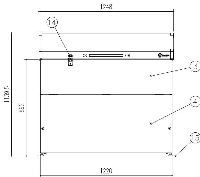
正面立面図
