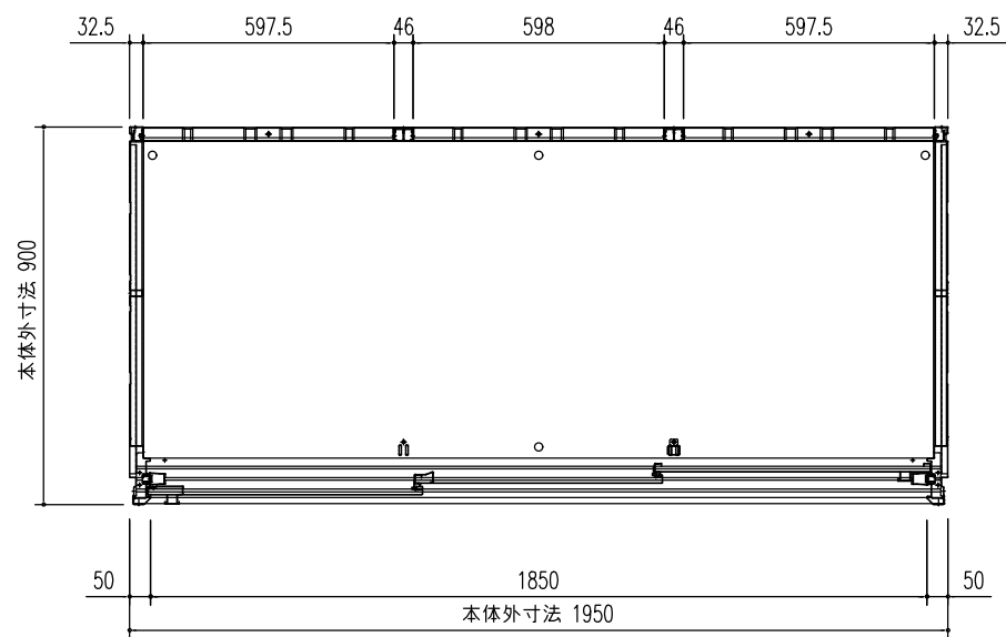
平面図 (S=1/20)
