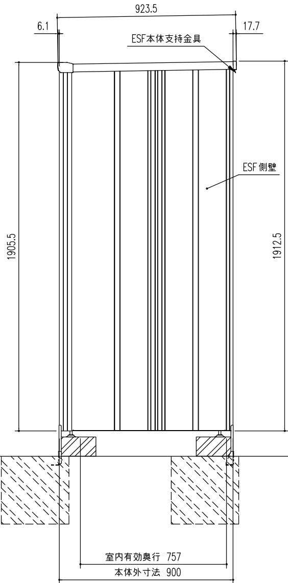
側面図 (S=1/20)
