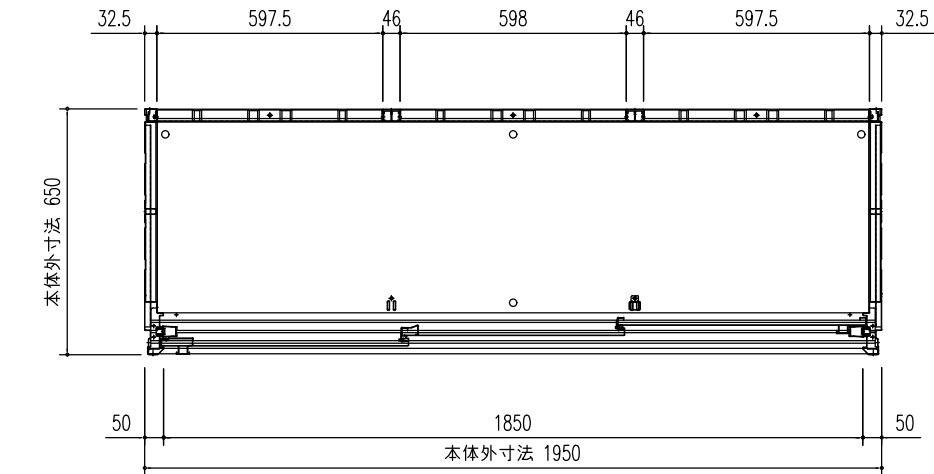
平面図 (S=1/20)
