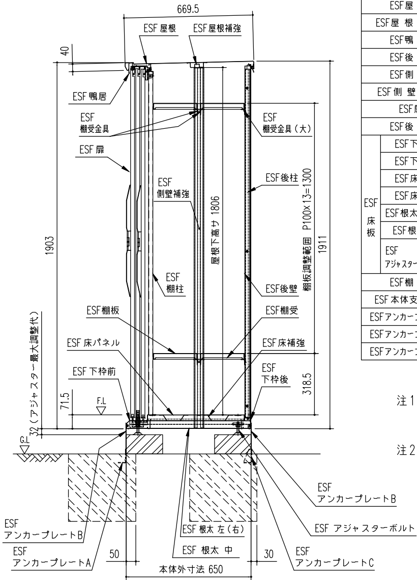
矩計図 (S=1/20)
