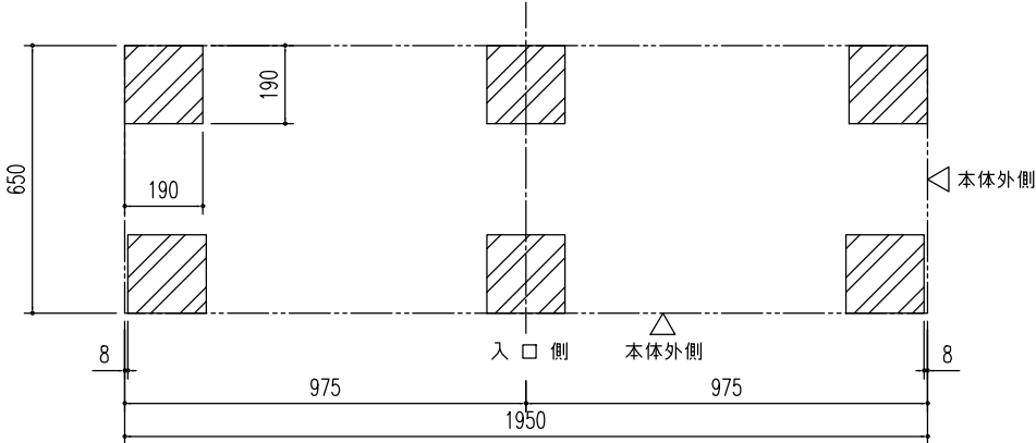
ブロック基礎伏図 (S=1/20)
