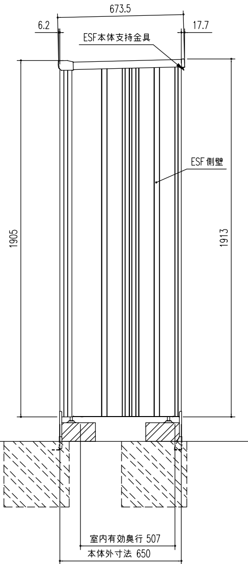
側面図 (S=1/20)
