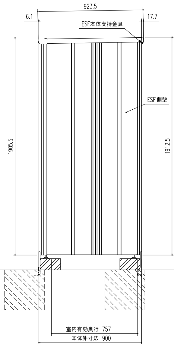
側面図 (S=1/20)
