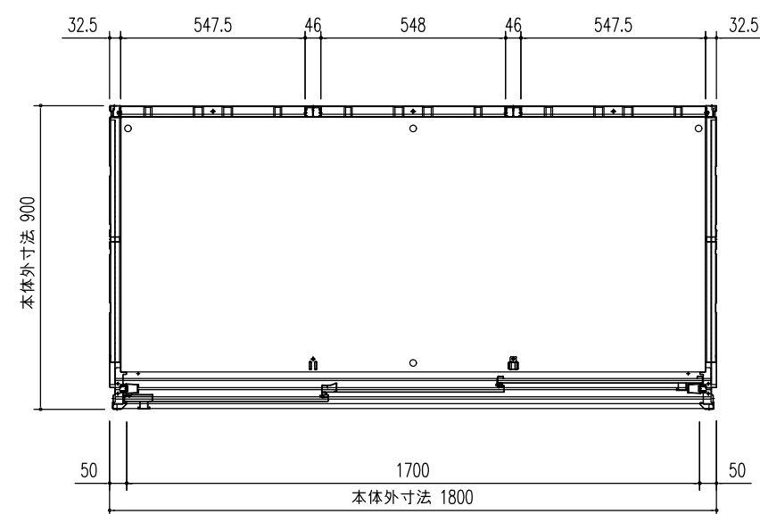
平面図 (S=1/20)
