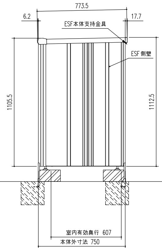
側面図 (S=1/20)
