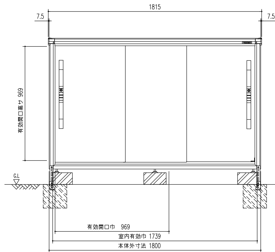
正面立面图 (S=1/20)
