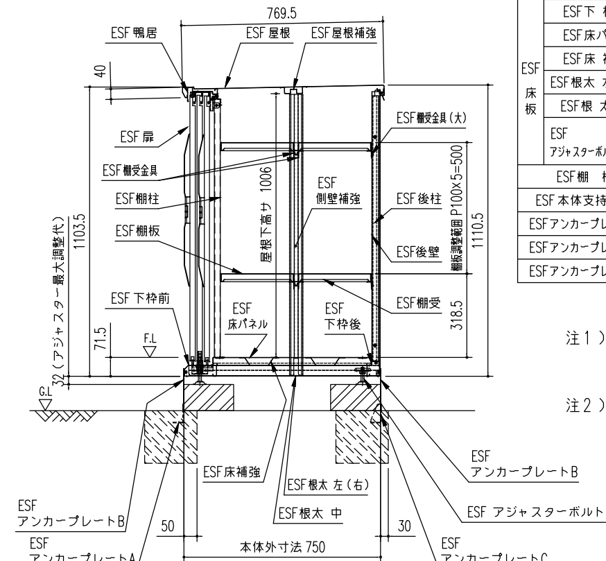
矩 計 図 ( S=1/20 )
