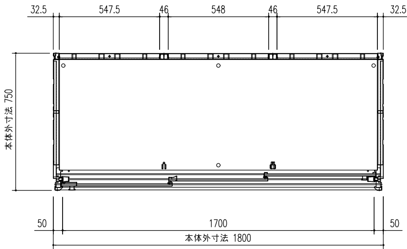
平面図 (S=1/20)
