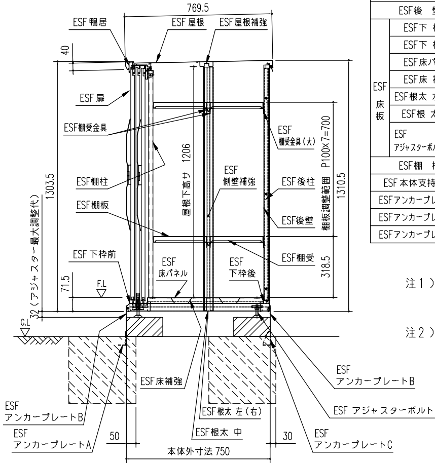
矩計図 (S=1/20)
