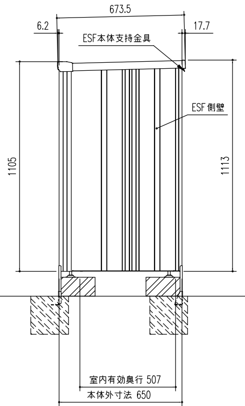
側面図 (S=1/20)
