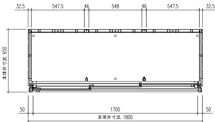
平面図 (S=1/20)
