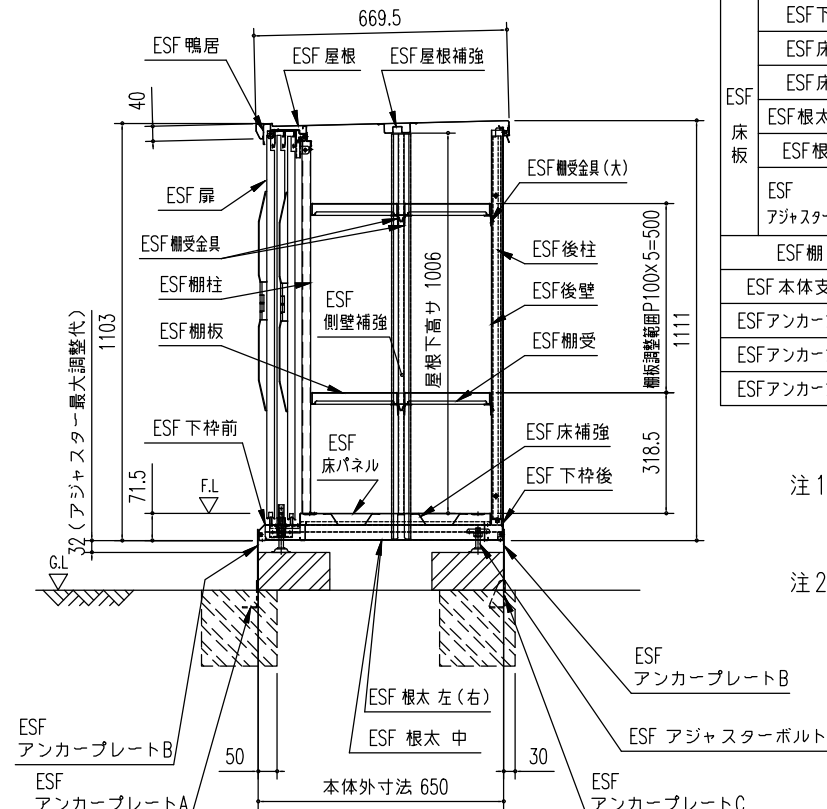
矩計図 (S=1/20)
