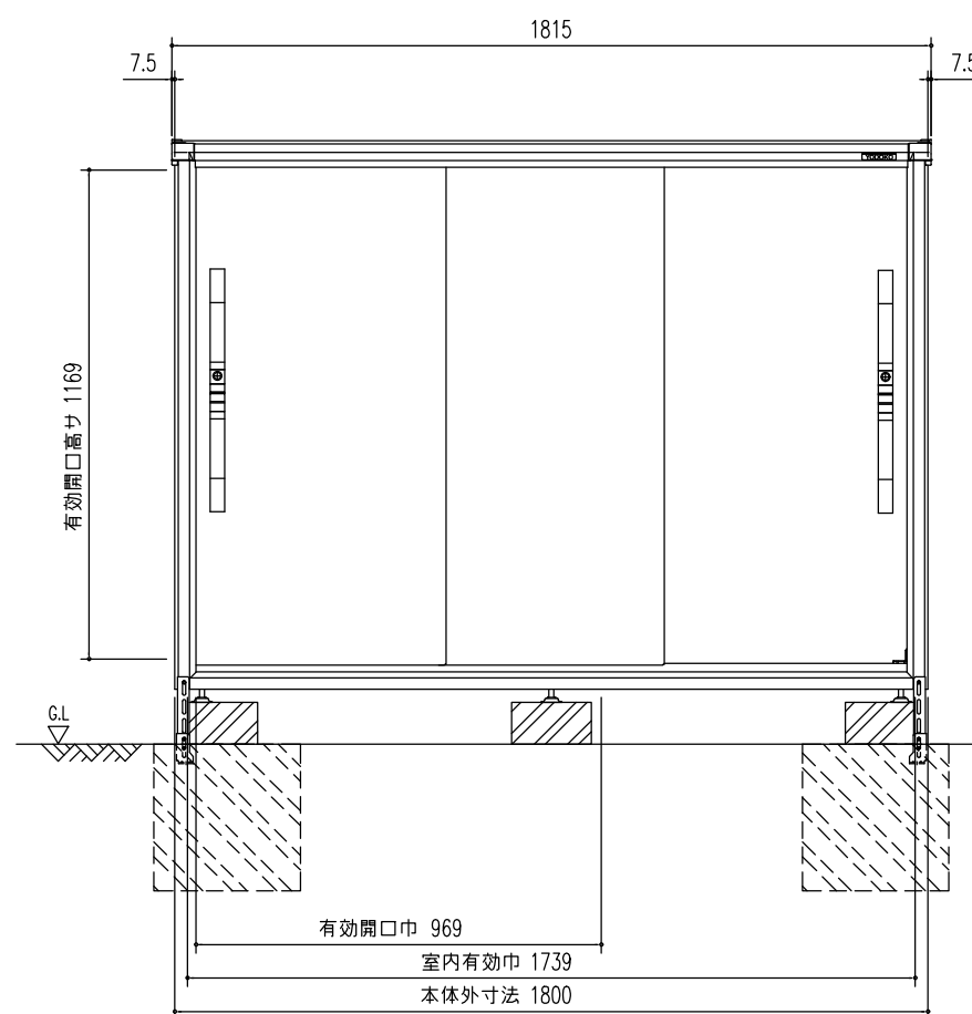
正面立面图 (S=1/20)
