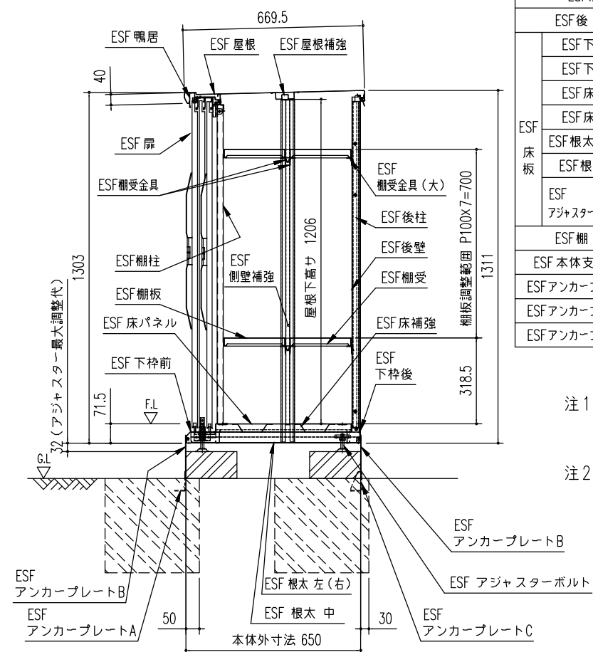
矩 計 図 (S=1/20)
