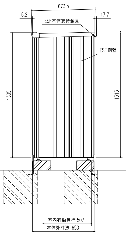
側面図 (S=1/20)
