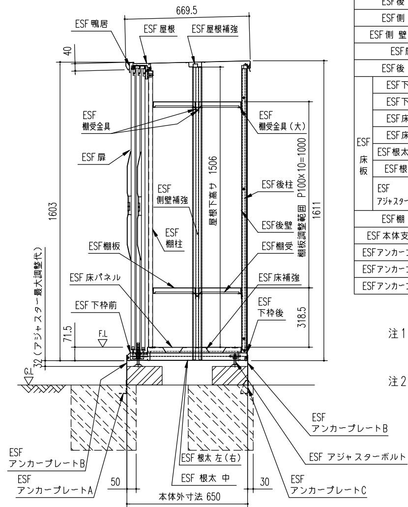
矩計図 (S=1/20)
