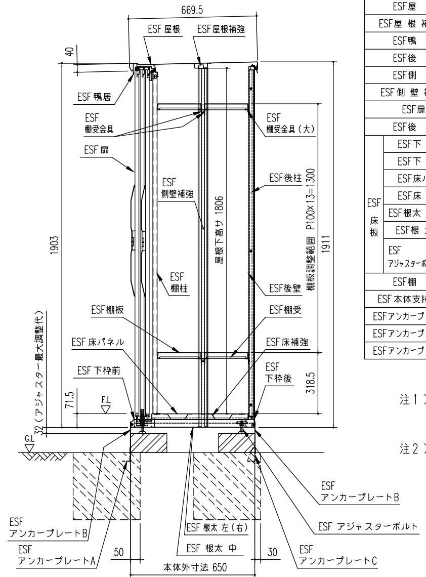
矩計図 (S=1/20)
