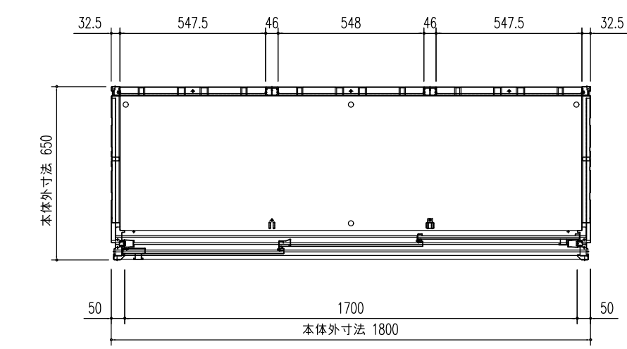
平面図 (S=1/20)
