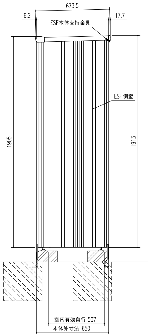
側面図 (S=1/20)
