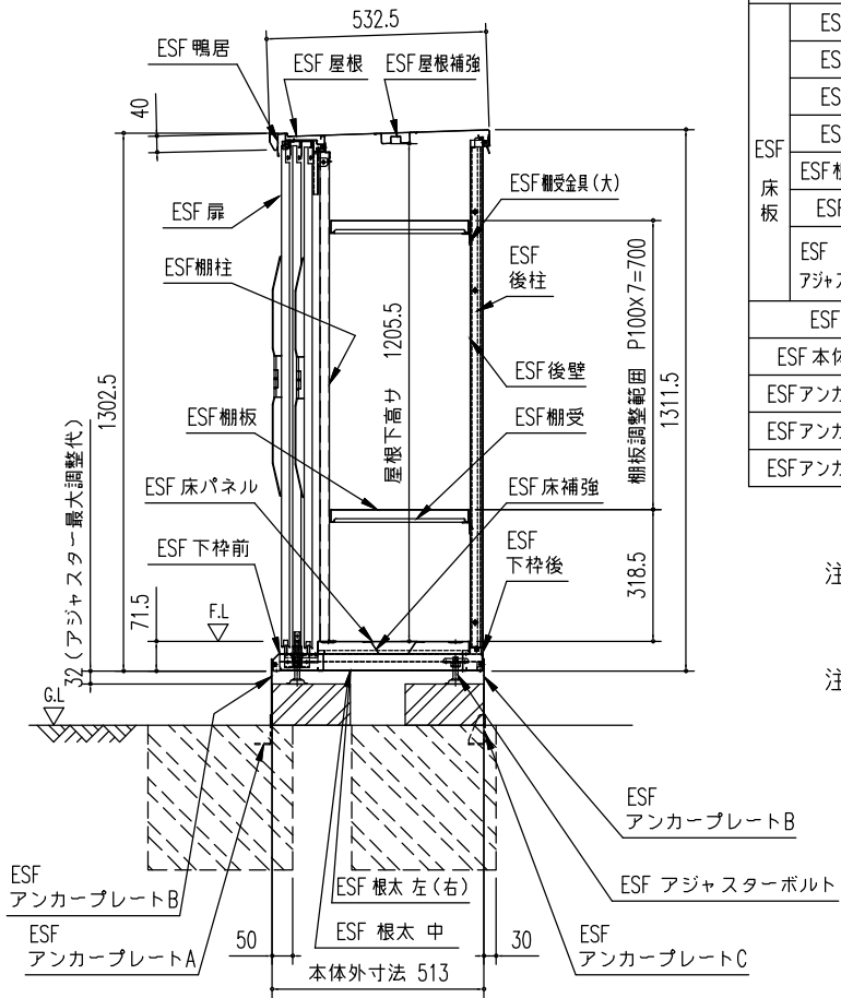
矩計図 (S=1/20)
