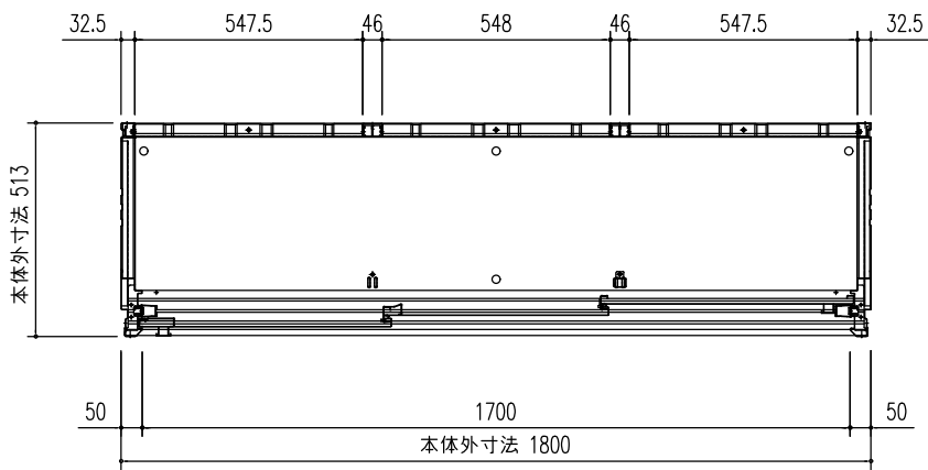
平面図 (S=1/20)
