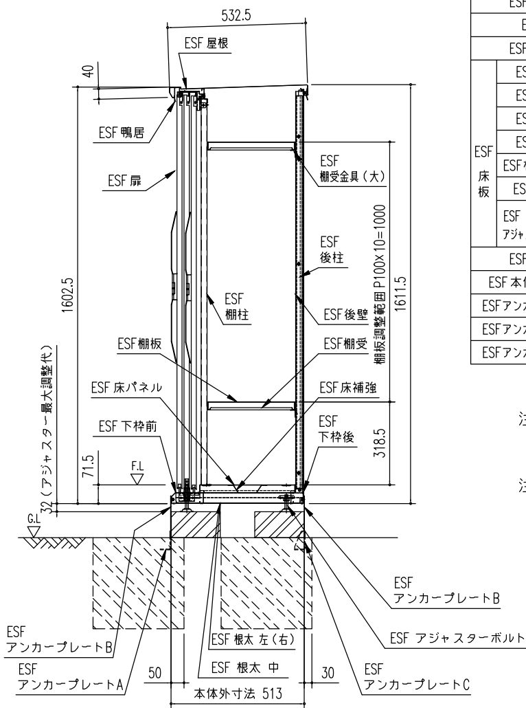
矩計図 (S=1/20)
