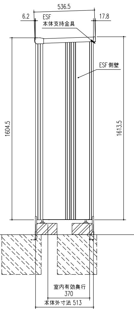
側面図 (S=1/20)
