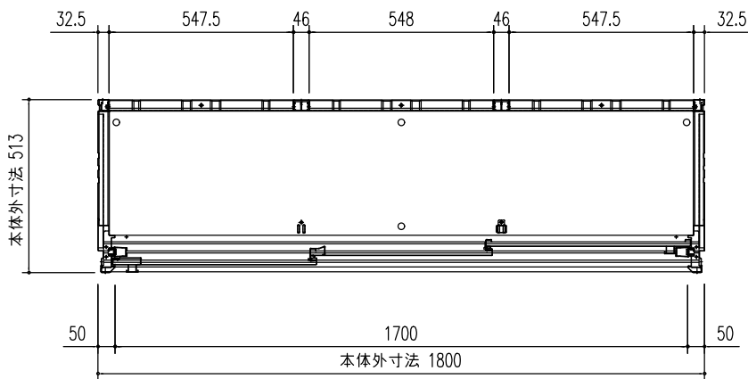
平面図 (S=1/20)
