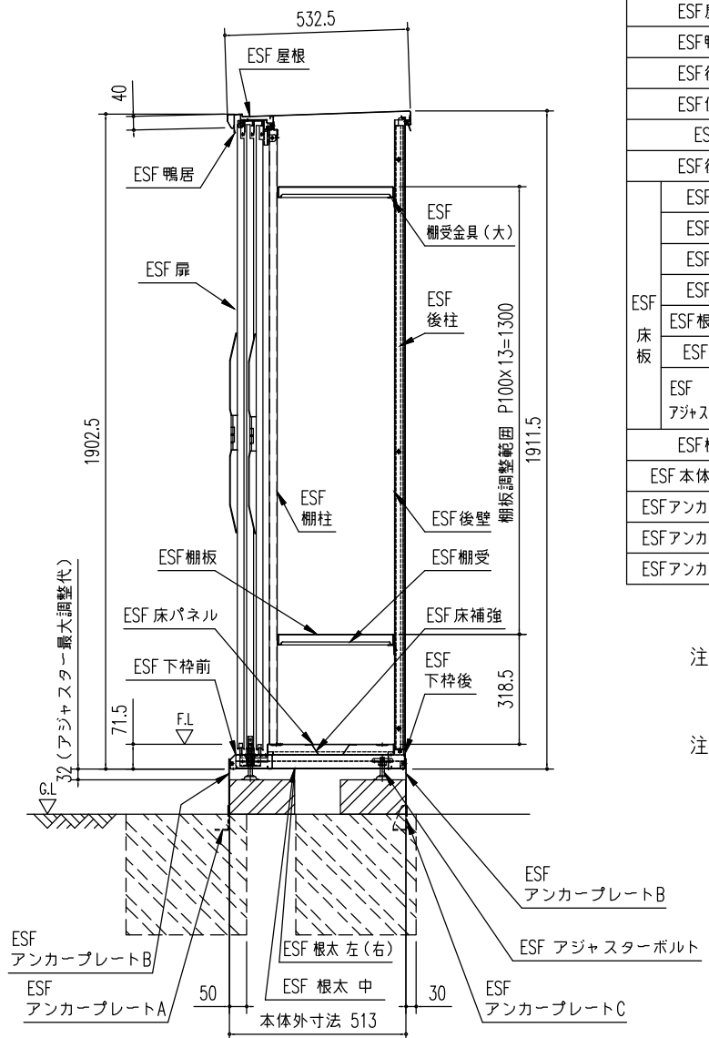
矩計図 (S=1/20)
