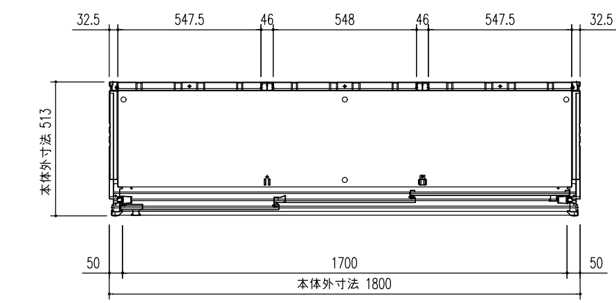
平面図 (S=1/20)
