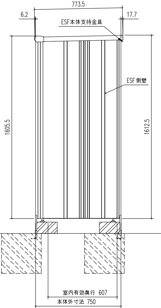
側面図 (S=1/20)
