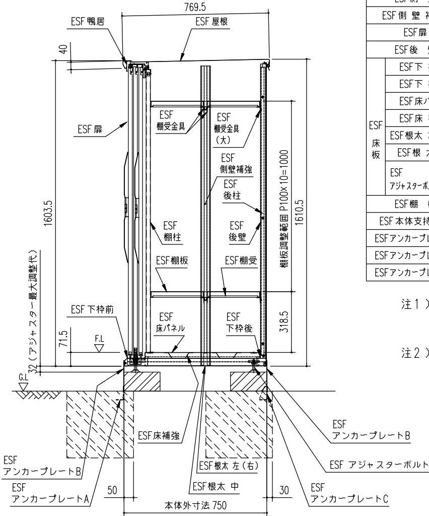
矩計図 (S=1/20)
