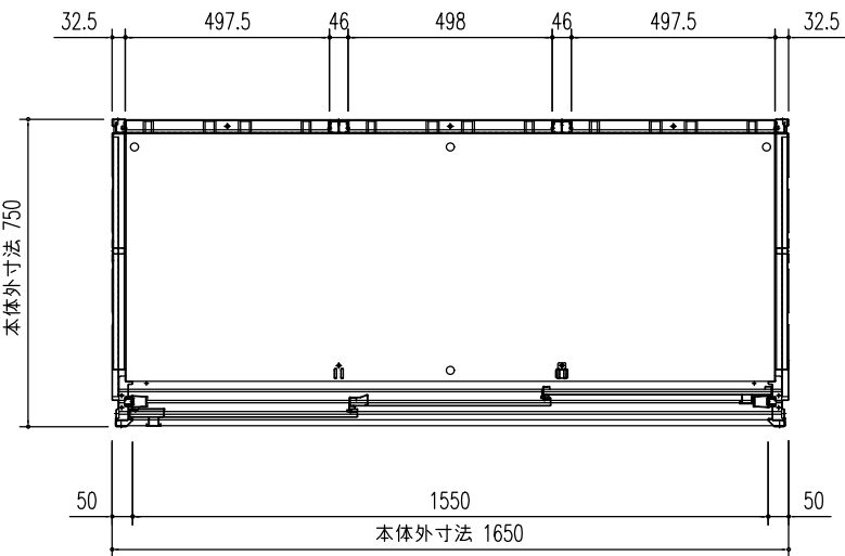
平面図 (S=1/20)
