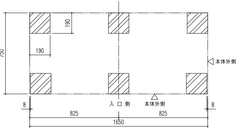
ブロック基礎伏図 (S=1/20)
