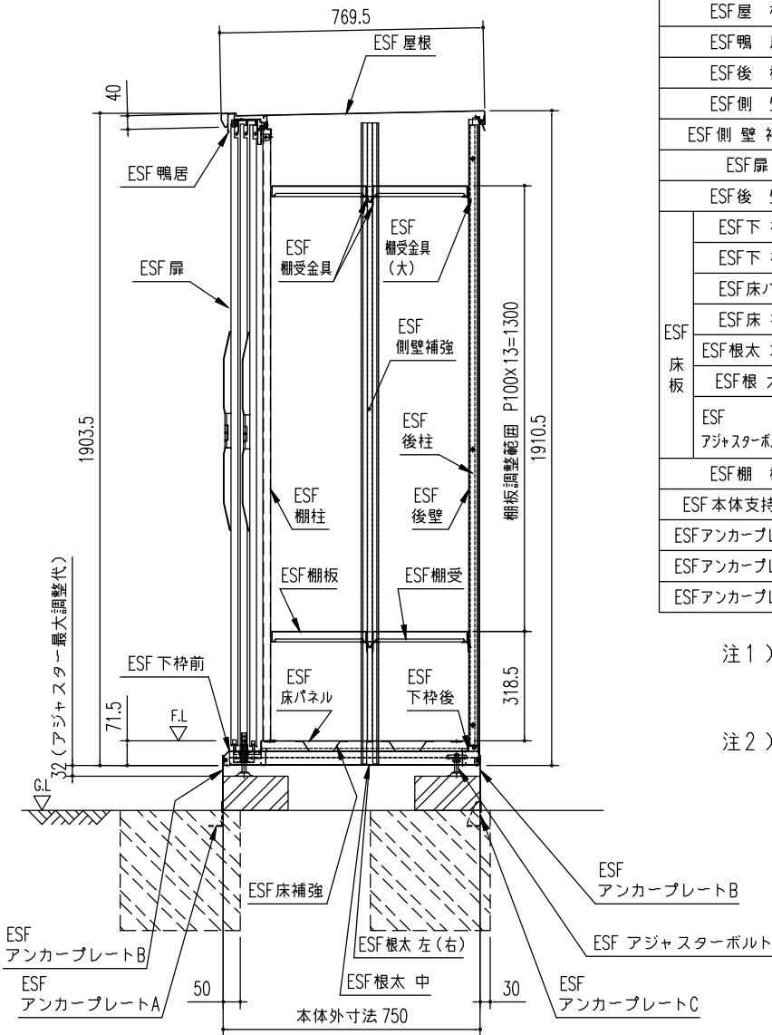
矩計図 (S=1/20)
