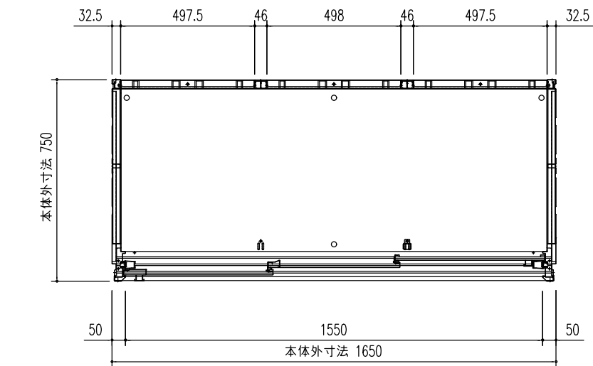
平面図 (S=1/20)
