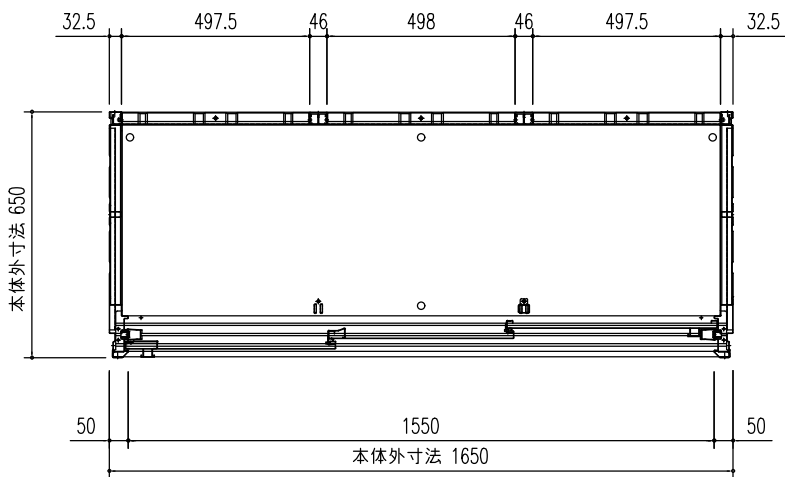
平面図 (S=1/20)
