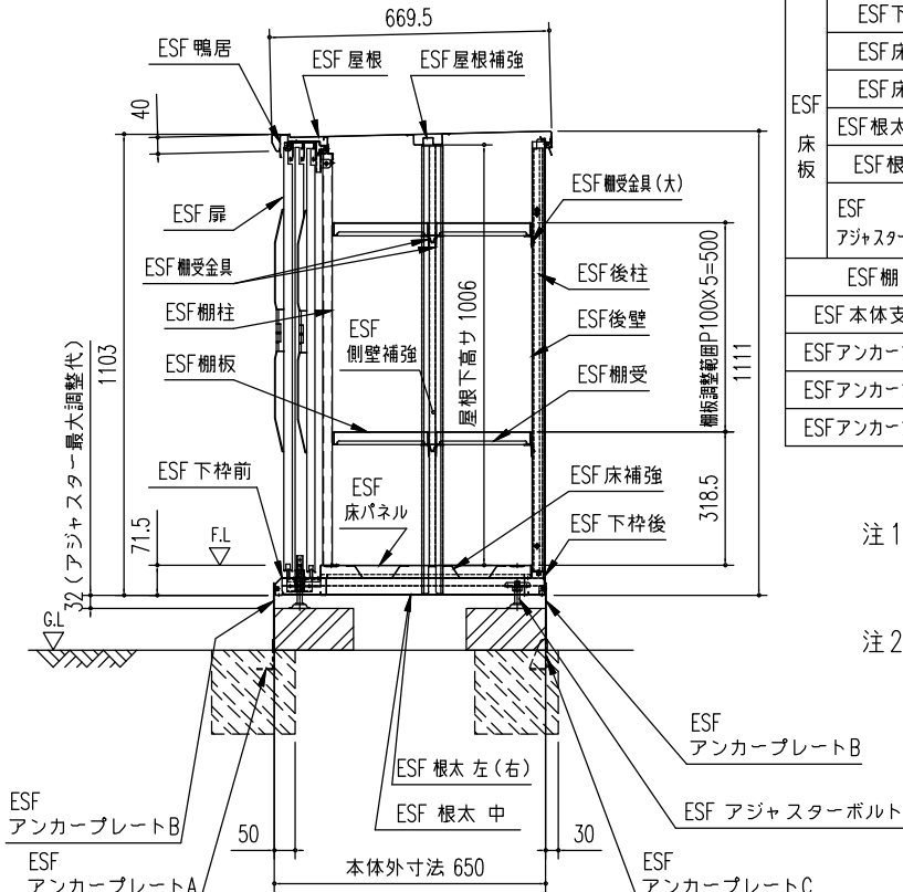
矩計図 (S=1/20)
