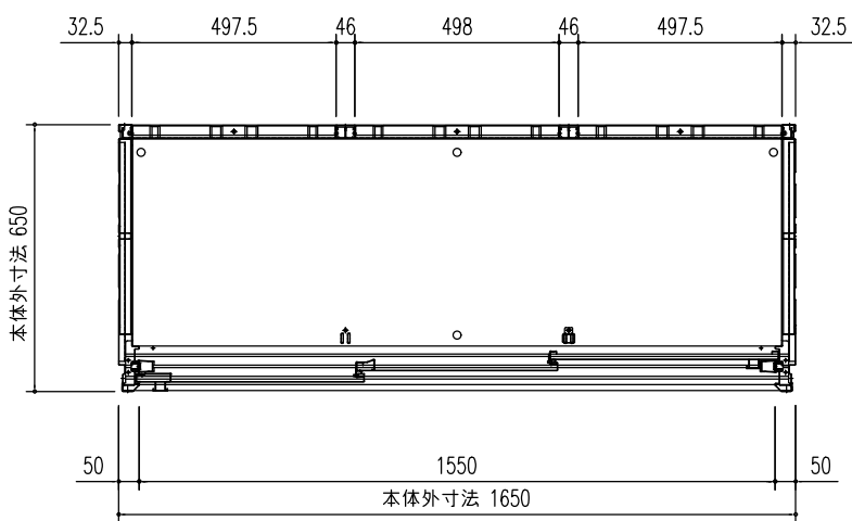
平面図 (S=1/20)
