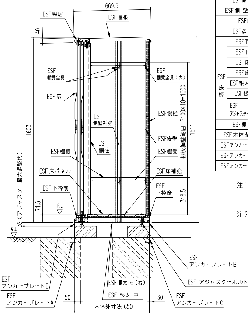
矩計図 (S=1/20)
