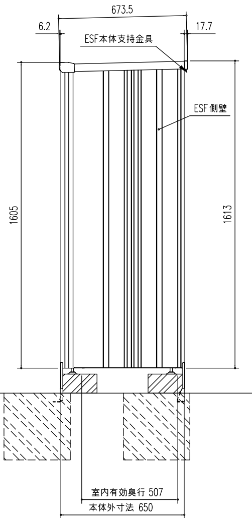
側面図 (S=1/20)
