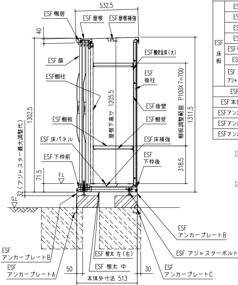
矩計図 (S=1/20)
