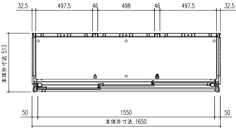
平面図 (S=1/20)
