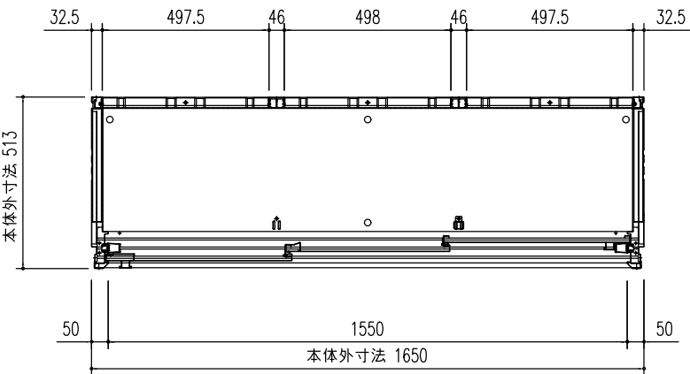
平面図 (S=1/20)
