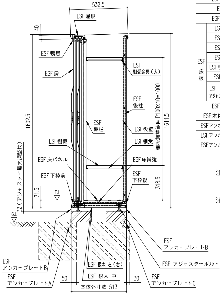
矩計図 (S=1/20)
