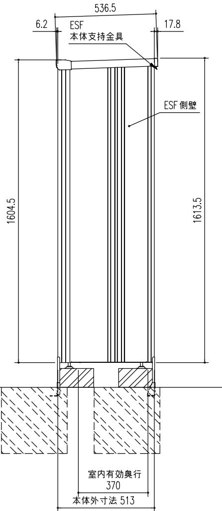
側面図 (S=1/20)
