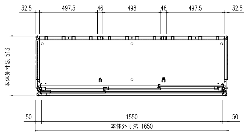
平面図 (S=1/20)
