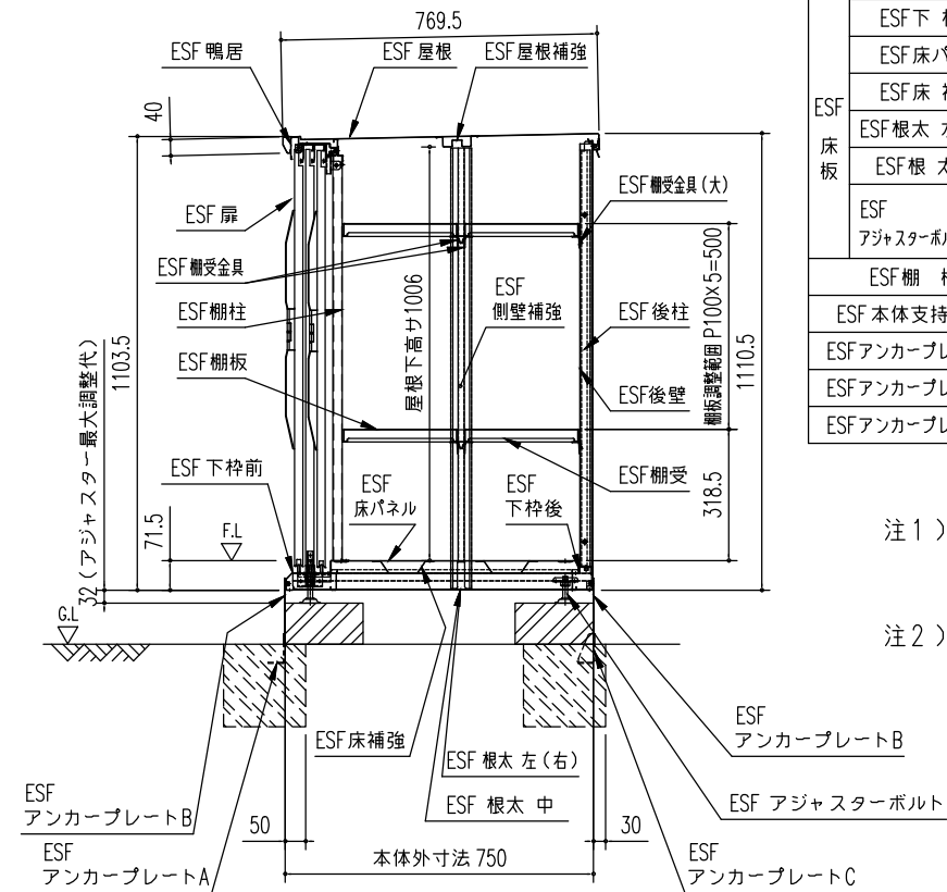
矩 計 図 ( S=1/20 )
