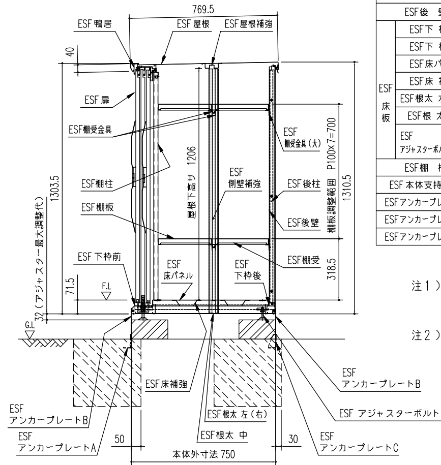
矩計図 (S=1/20)
