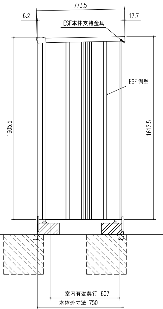
側面図 (S=1/20)
