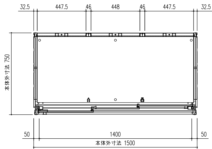
平面図 (S=1/20)
