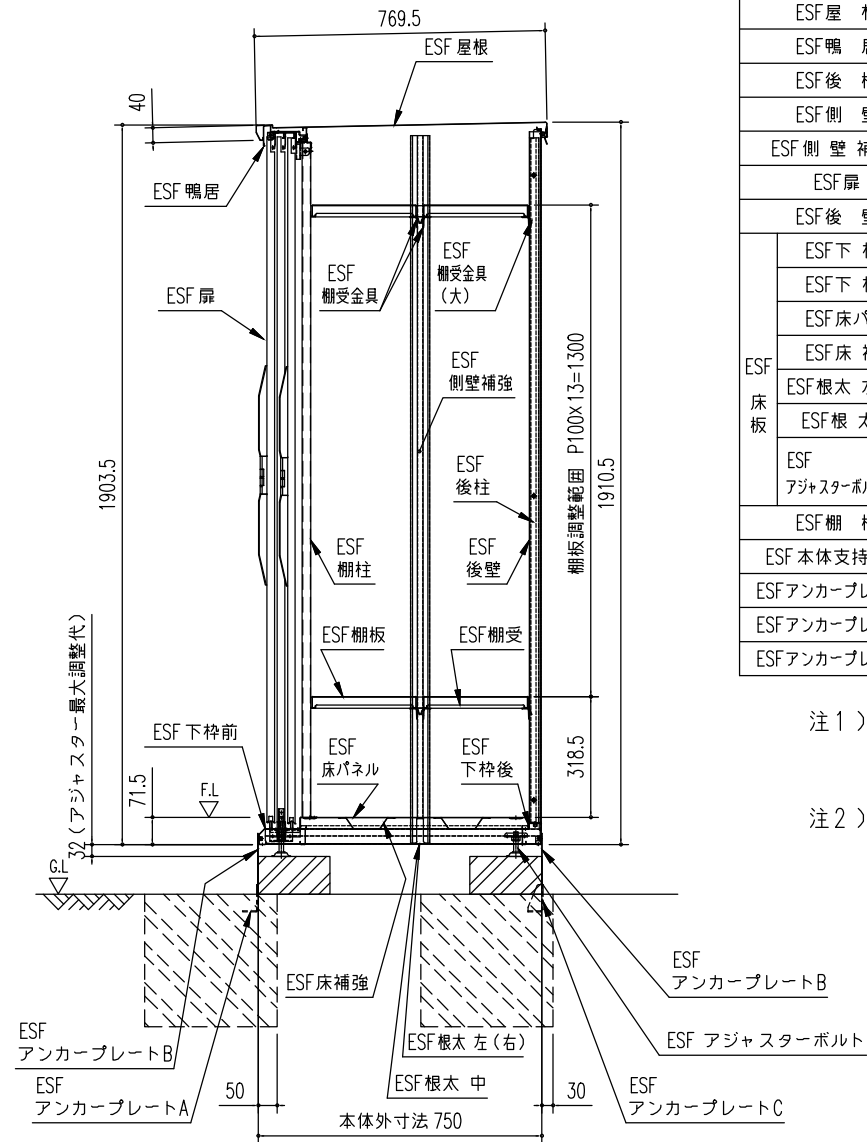
矩計図 (S=1/20)
