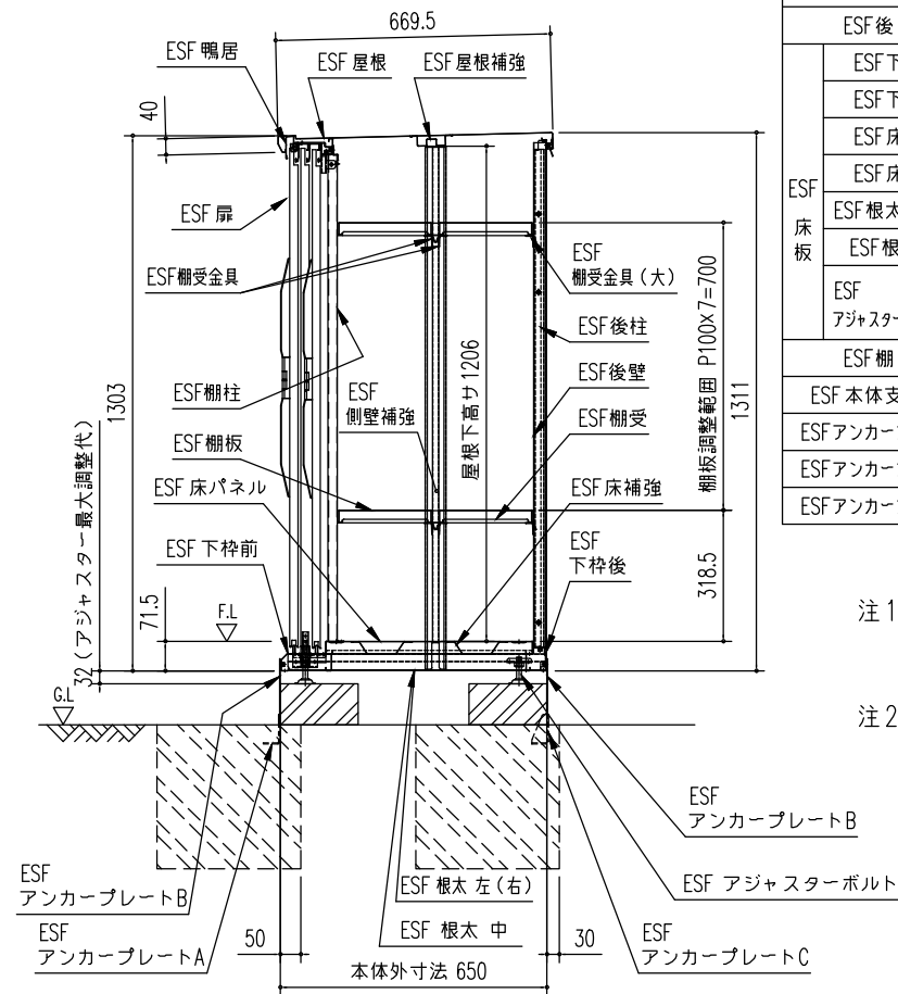
矩計図 (S=1/20)
