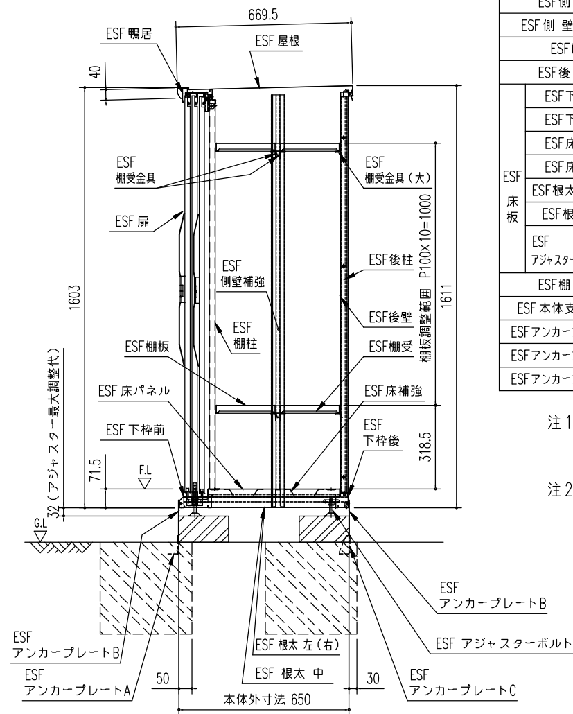
矩計図 (S=1/20)
