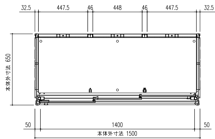
平面図 (S=1/20)
