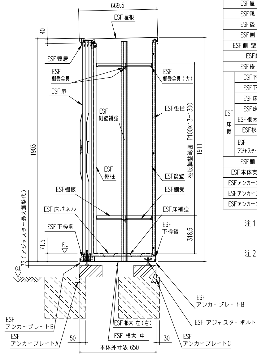
矩計図 (S=1/20)
