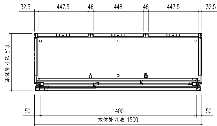
平面図 (S=1/20)
