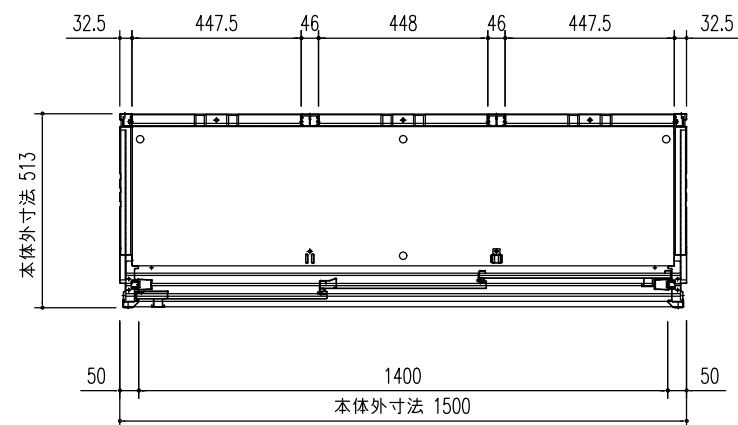
平面図 (S=1/20)
