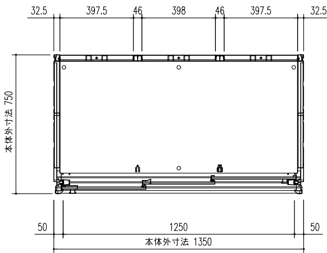
平面図 (S=1/20)
