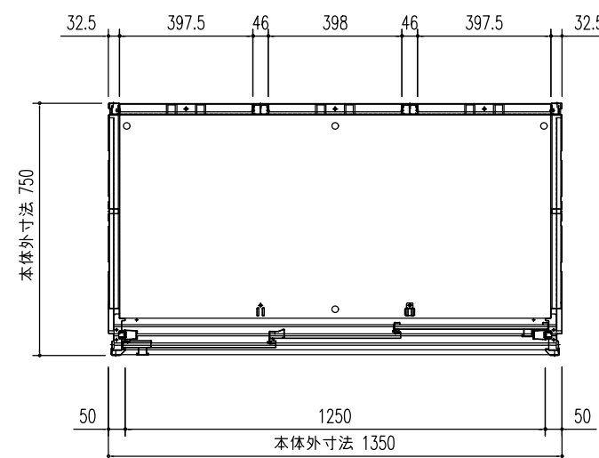
平面図 (S=1/20)
