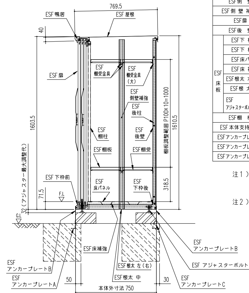
矩 計 図 (S=1/20)
