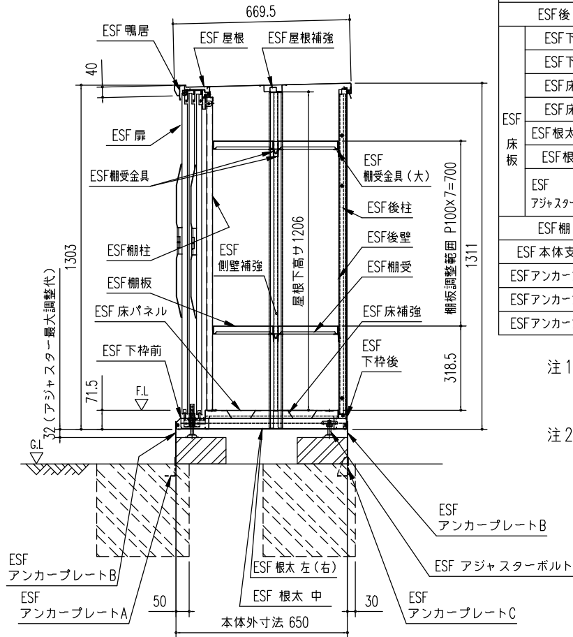
矩計図 (S=1/20)
