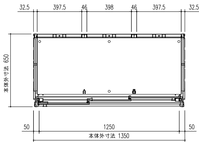
平面図 (S=1/20)
