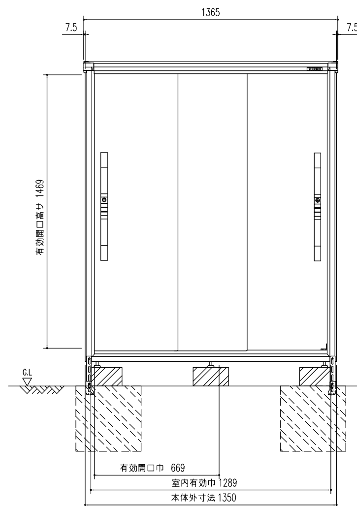
正面立面图 (S=1/20)
