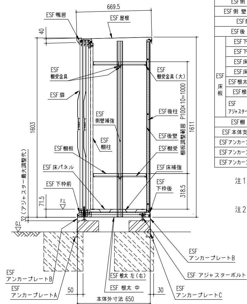
矩 計 図 (S=1/20)
