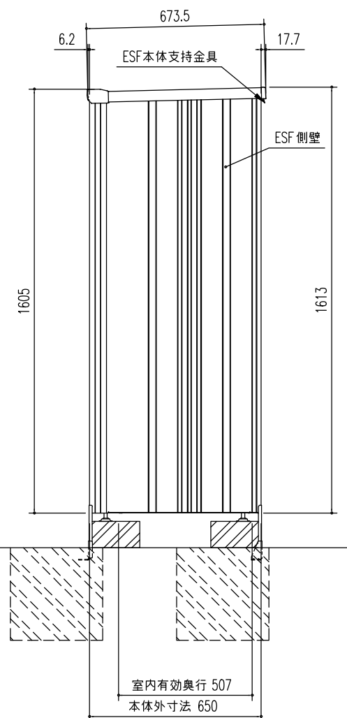
側 面 図 (S=1/20)
