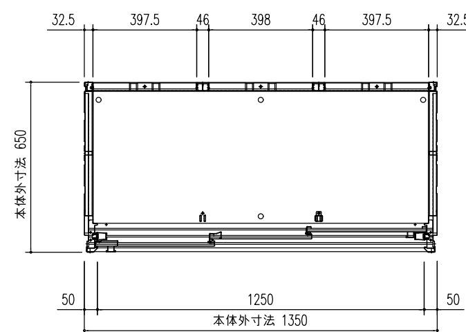
平面図 (S=1/20)
