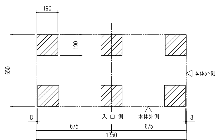
ブロック基礎伏図 (S=1/20)
