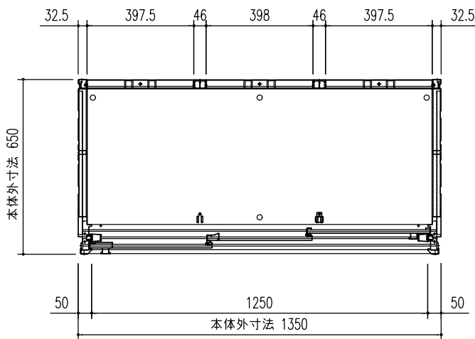
平面図 (S=1/20)
