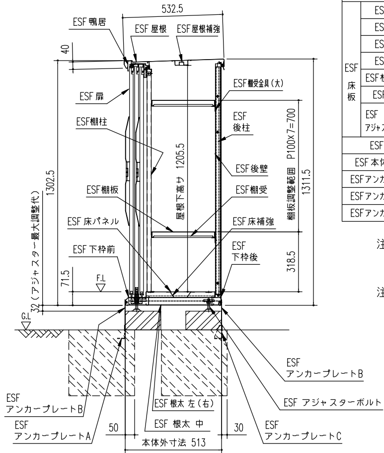
矩計図 (S=1/20)
