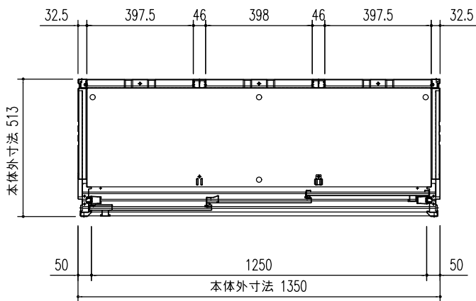
平面図 (S=1/20)
