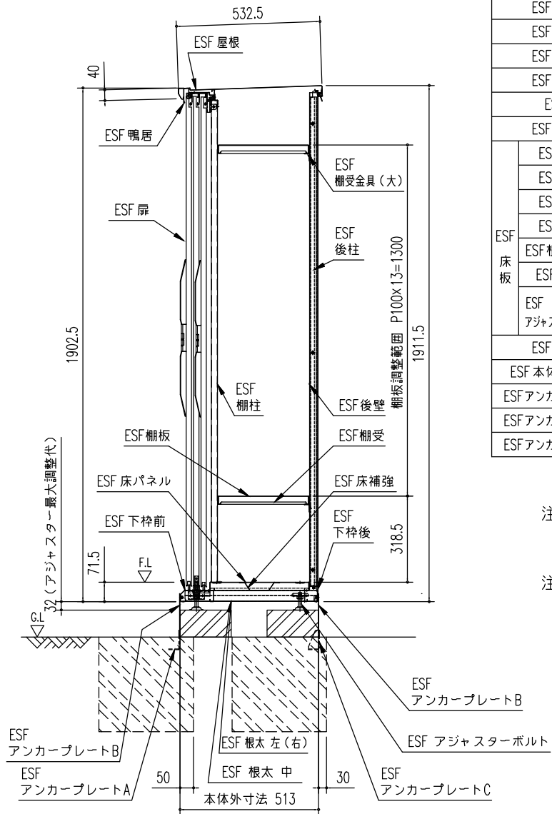
矩計図 (S=1/20)
