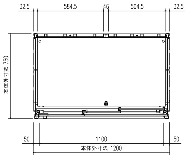
平面図 (S=1/20)
