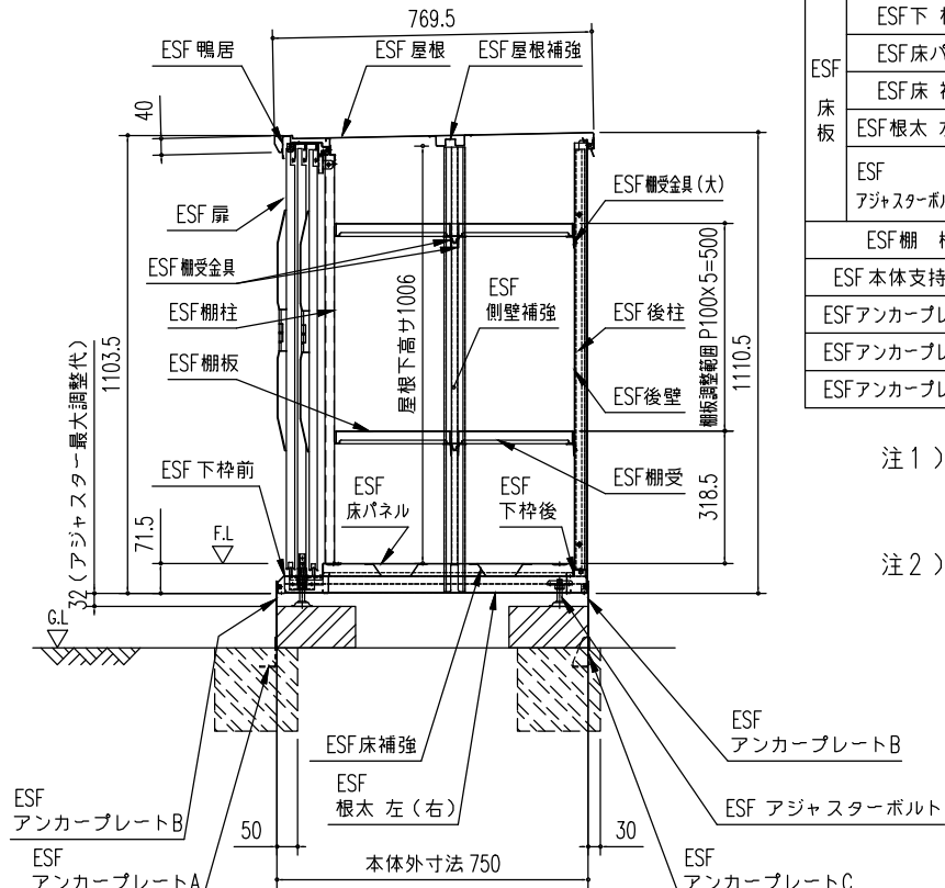
矩計図 (S=1/20)
