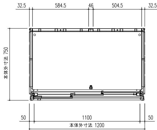
平面図 (S=1/20)
