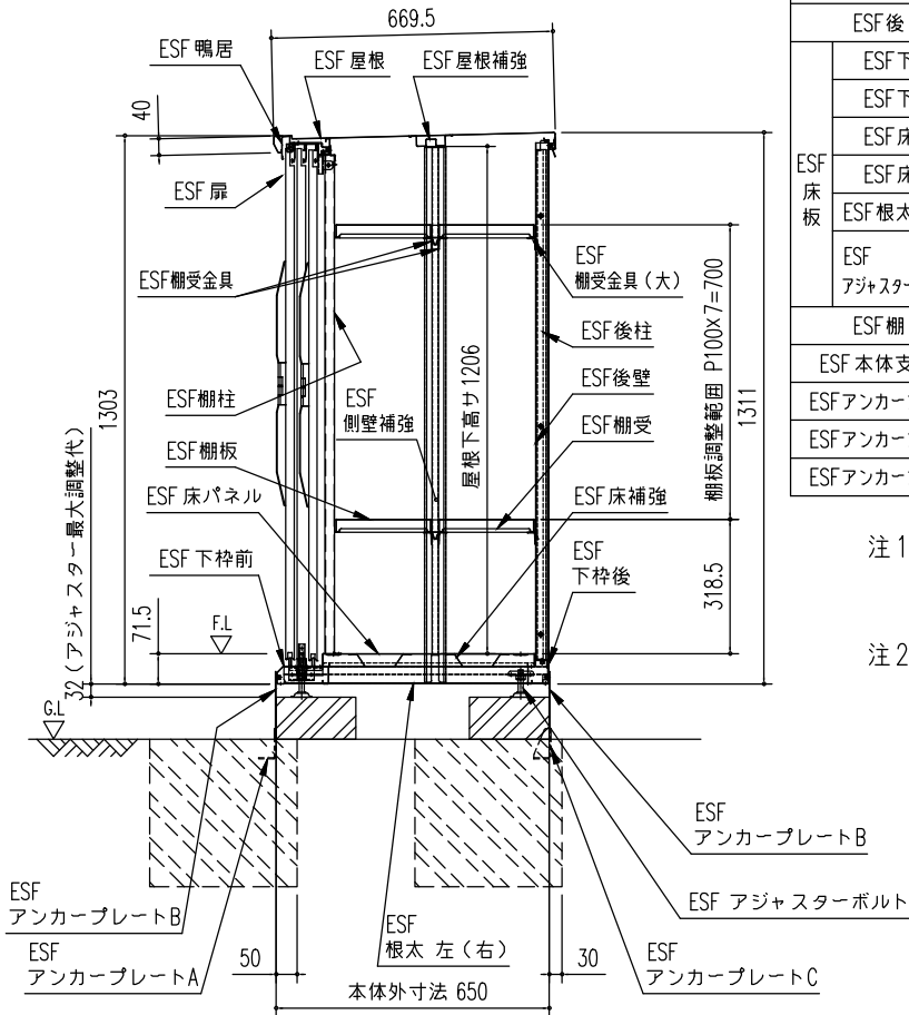
矩計図 (S=1/20)
