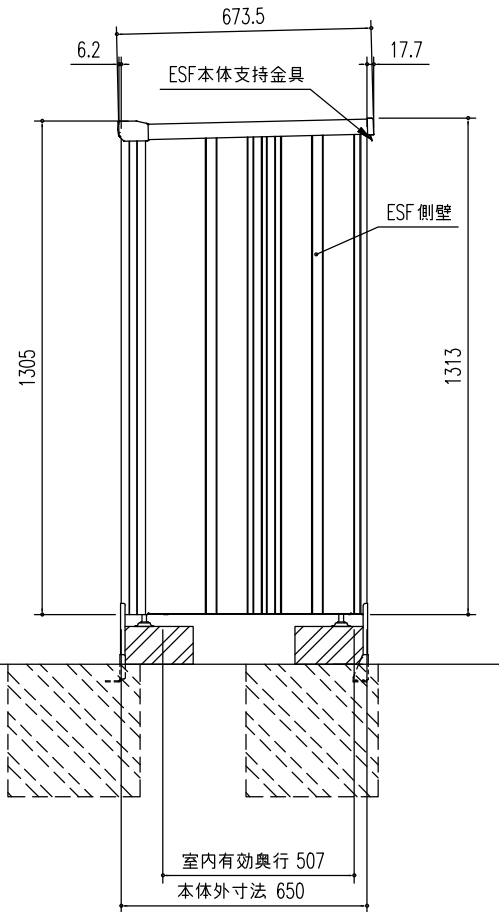
側面図 (S=1/20)
