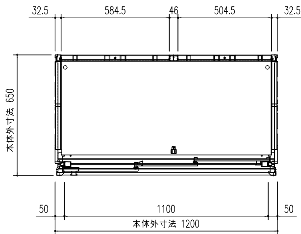
平面図 (S=1/20)
