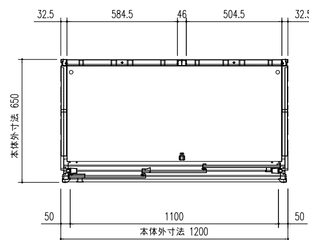
平面図 (S=1/20)
