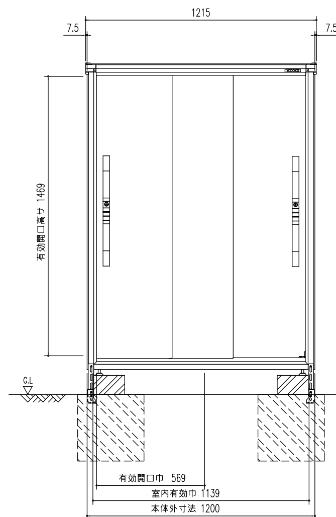
正 面 立 面 图 (S=1/20)
