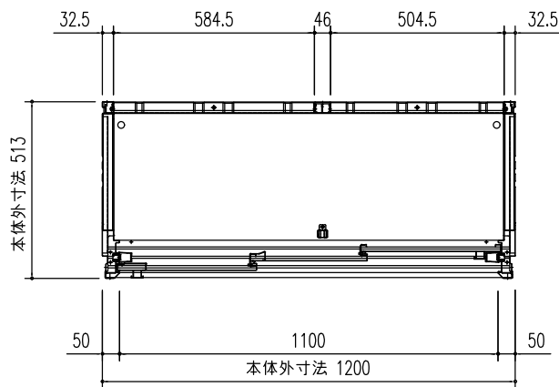
平面図 (S=1/20)
