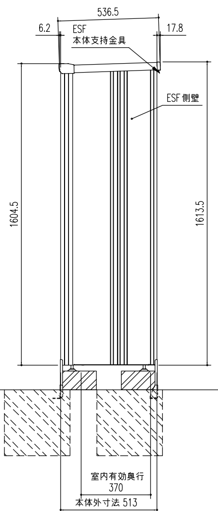
側 面 図 (S=1/20)
