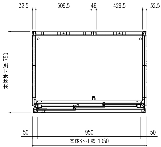
平面図 (S=1/20)
