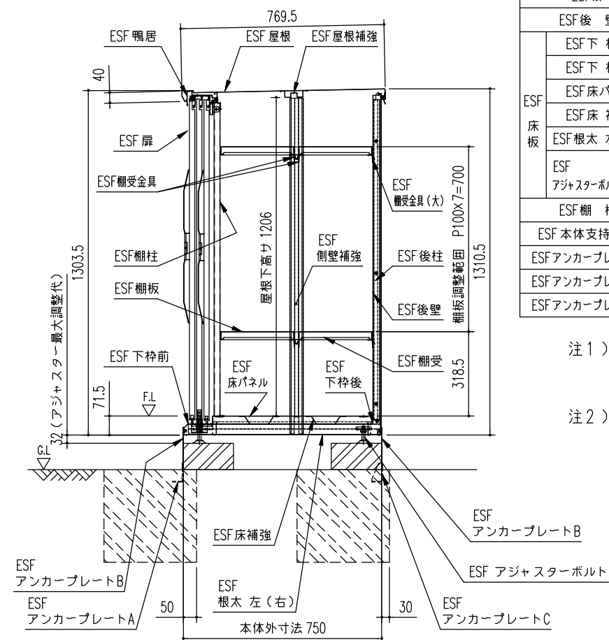
矩 計 図 (S=1/20)
