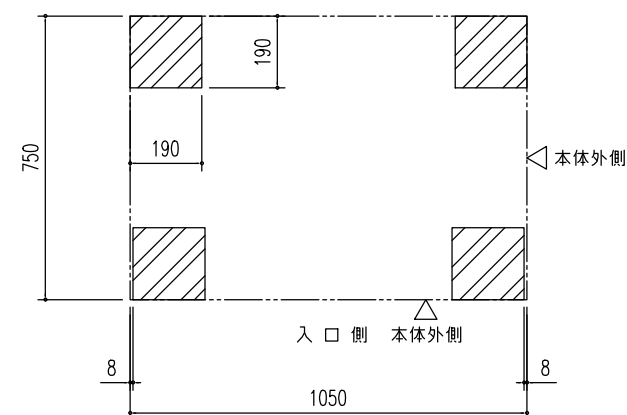
ブロック基礎伏図 (S=1/20)
