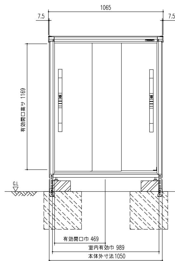
正面立面图 (S=1/20)
