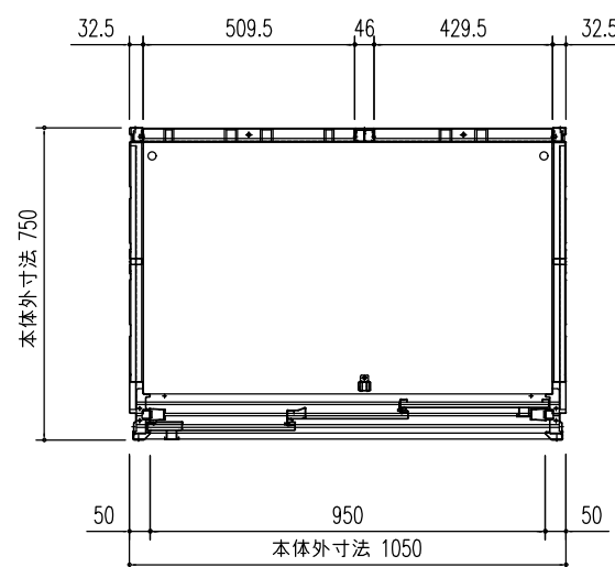
平面図 (S=1/20)
