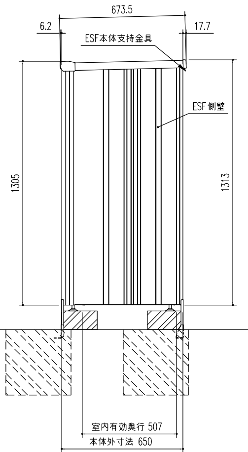
側面図 (S=1/20)
