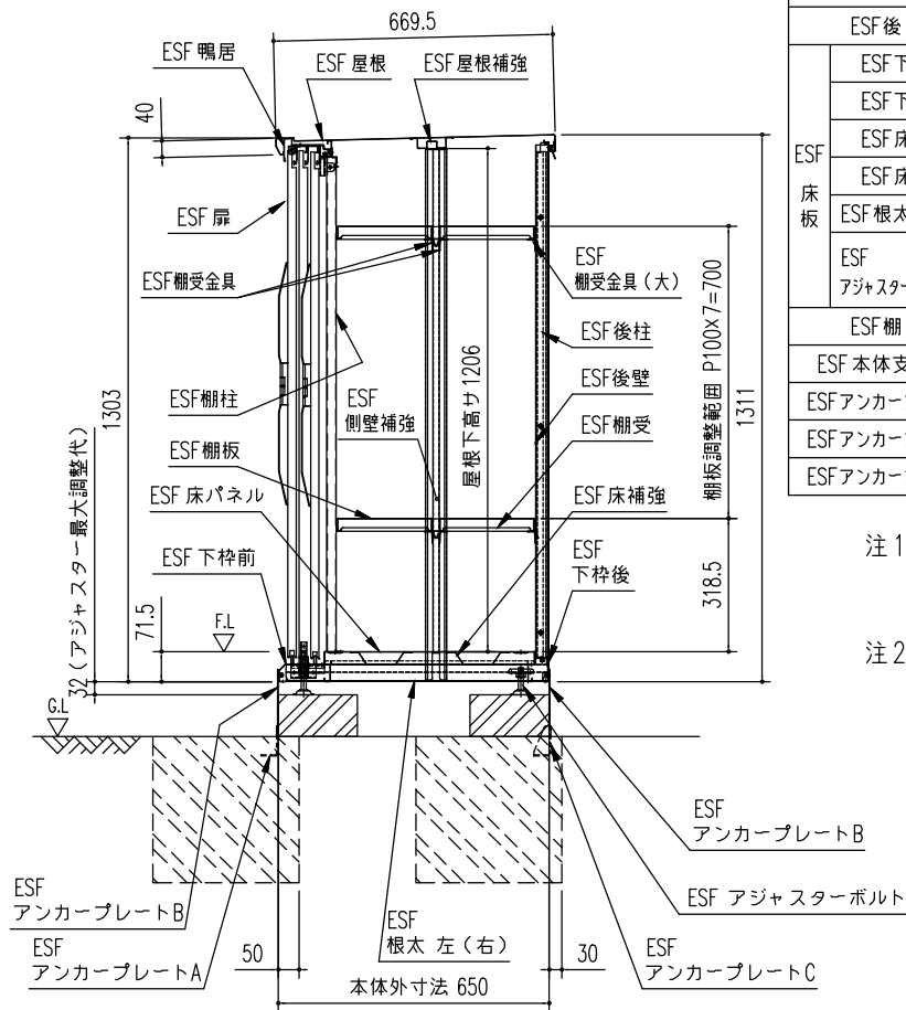
矩計図 (S=1/20)
