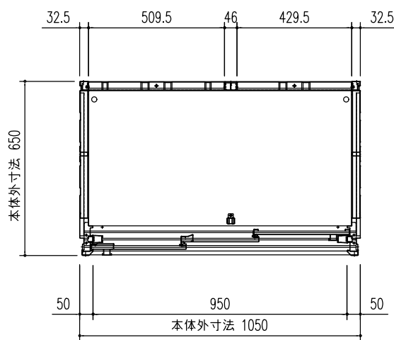
平面図 (S=1/20)
