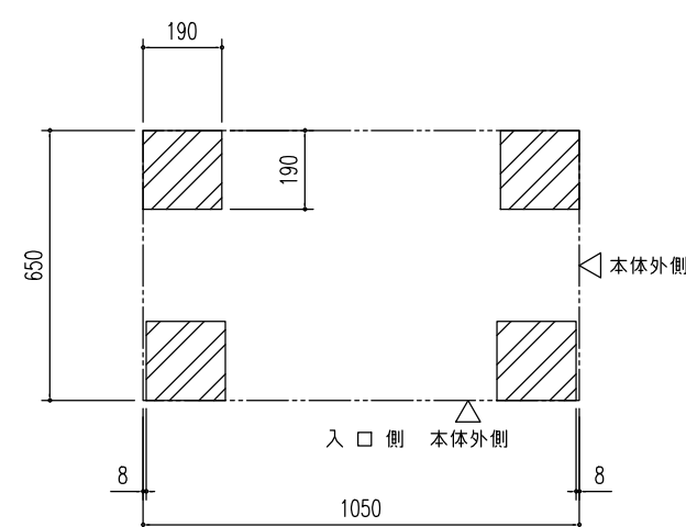
ブロック基礎伏図 (S=1/20)
