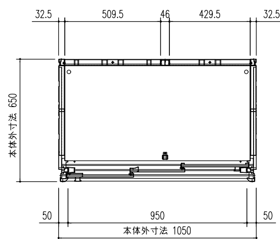
平面図 (S=1/20)
