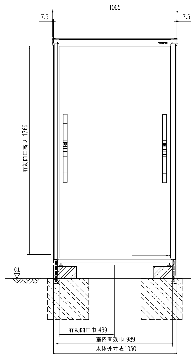
正面立面图 (S=1/20)
