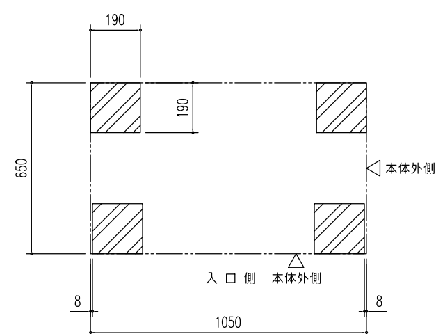
ブロック基礎伏図 ( S=1/20 )
