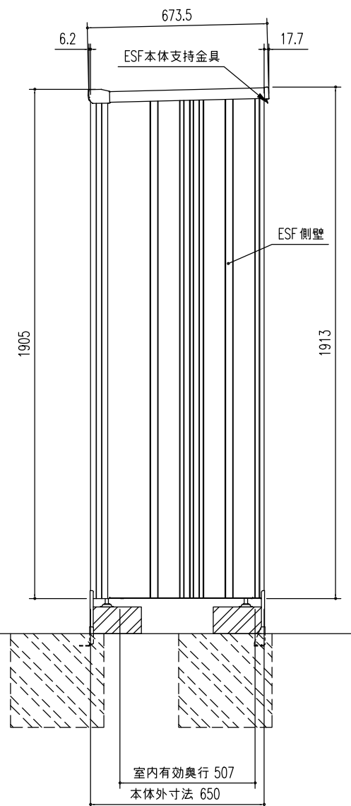
側 面 図 (S=1/20)
