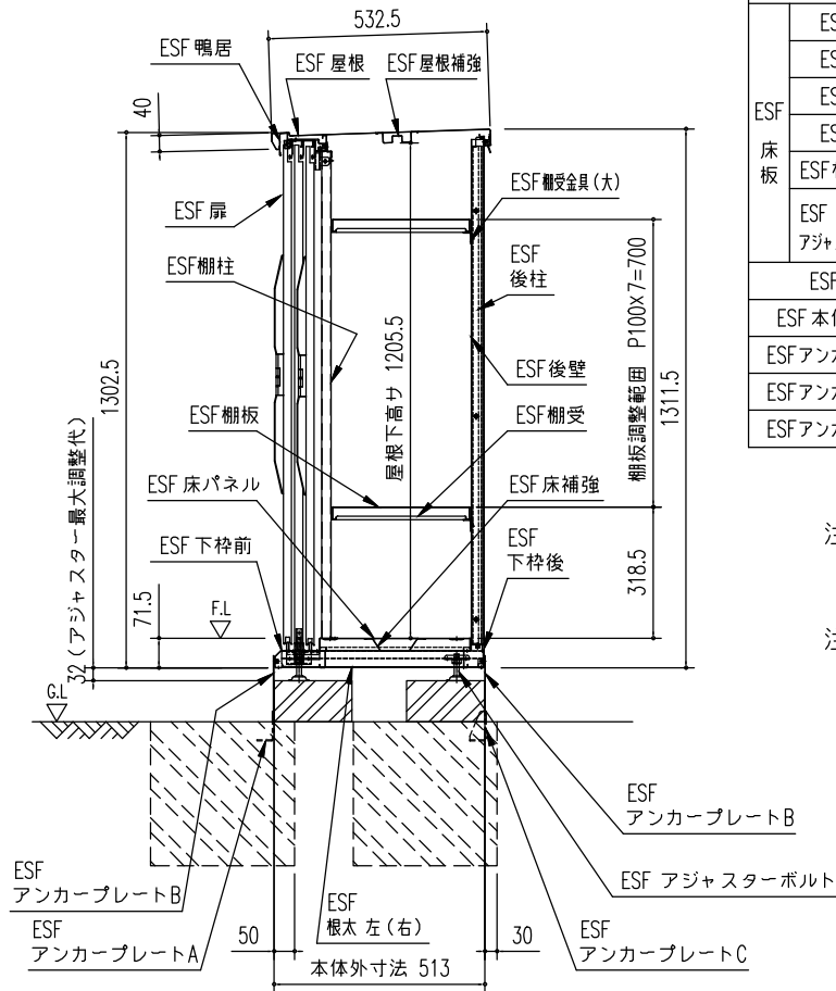
矩計図 (S=1/20)
