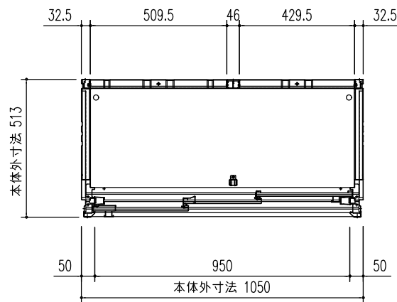
平面図 (S=1/20)
