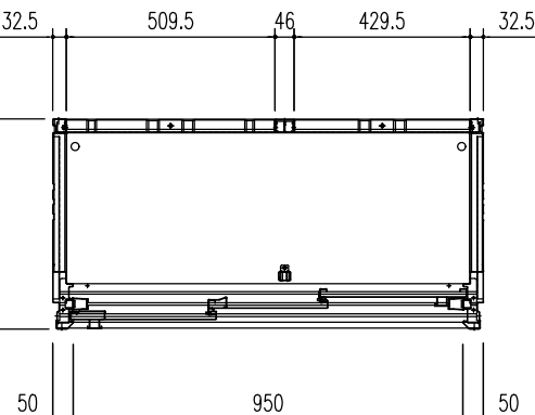
本体外寸法 1050
